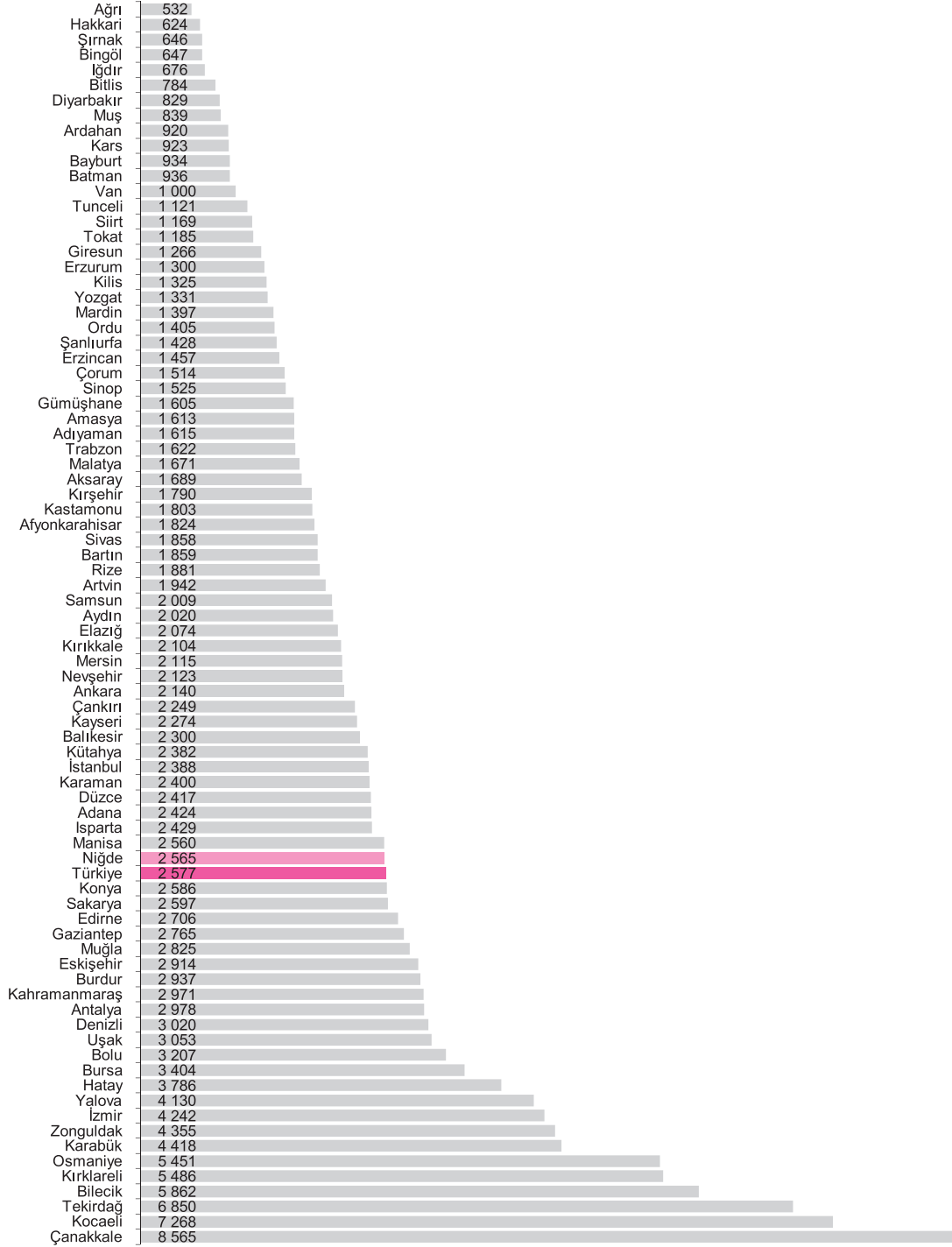
Grafik 1.24 Kişi başına toplam elektrik tüketimi, 2012 (KWh)
